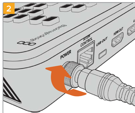
Sichern Sie die Kabelverbindung zum ATEM Mini, indem Sie den Verbinder am Gerät festziehen
